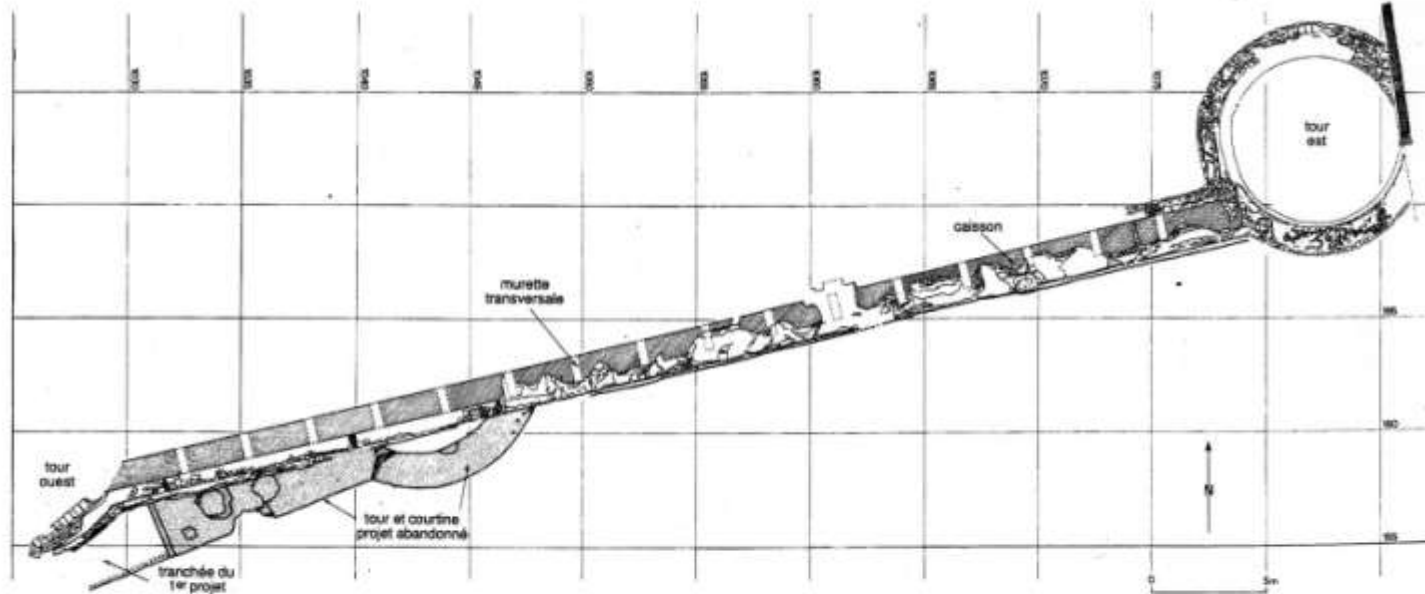
FIG. 7 — Plan des vestiges de l'enceinte à l'hôpital Larrey dégagés lors de l'opération archéologique.
