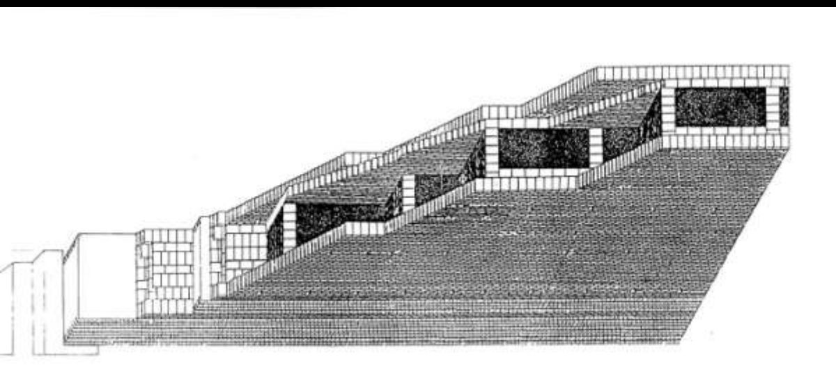
Fig. 15 — Schéma du système d'accrochage des murettes transversales du blocage avec les parements.
