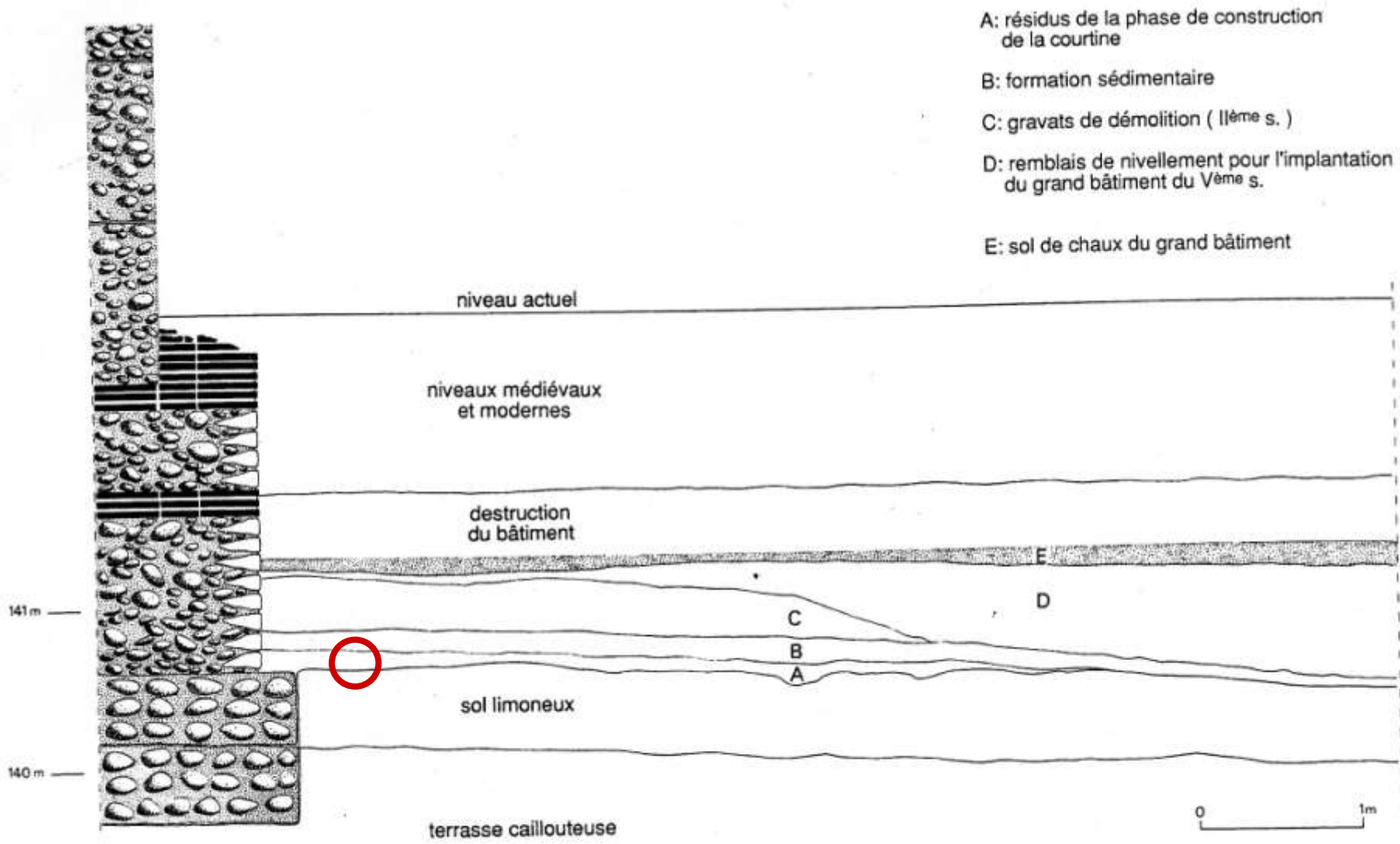
Fig. 8 — Coupe stratigraphique des niveaux accumulés au pied de la courtine, pendant et après sa construction : axe nord-sud 1055.
