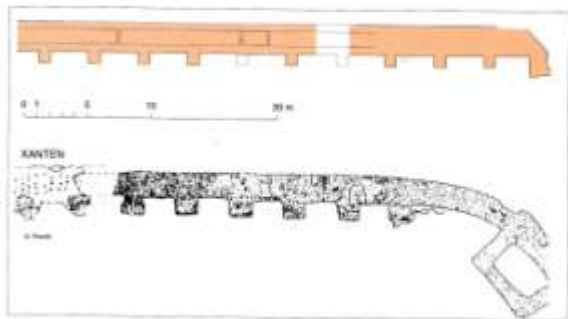
FIG. 219. PLAN DÉTAILLÉ DE LA PORTÉE À L'ENTRÉE OCCIDENTALE ET DE L'ENTRÉE DE KASBAH. D'après Alain Badi.
