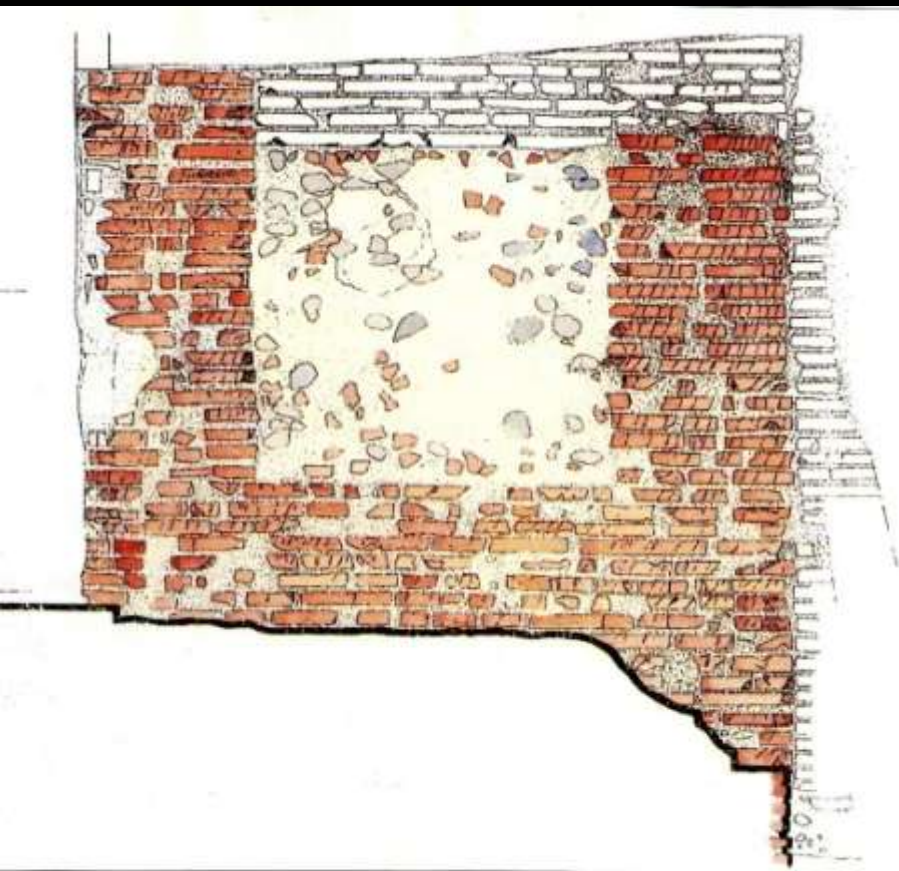
FIG. 162. REMPART DE L'INSTITUT CATHOLIQUE. COUPE DANS LE COULOIR DE SERVICE. Dessin P. Moly et A. el-Kandoussi.
