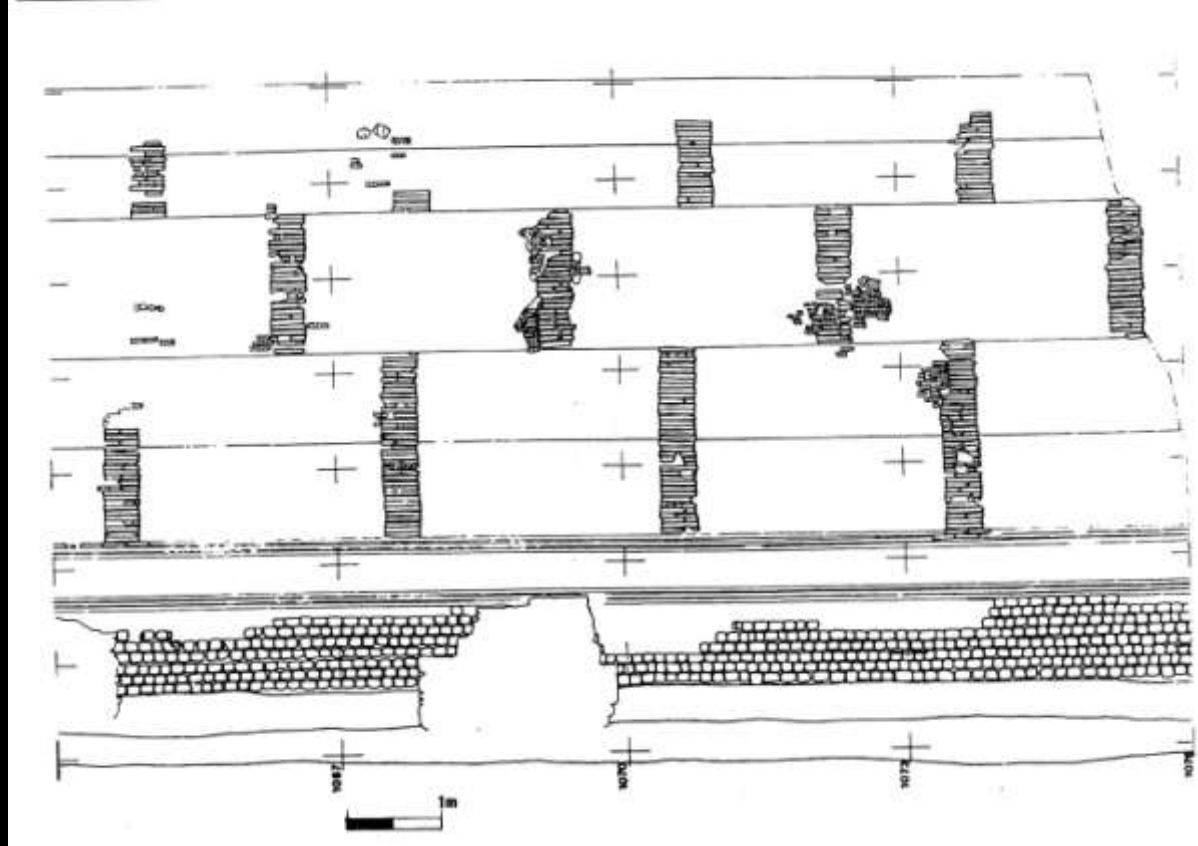
Fig. 15 — Schéma du système d'accrochage des murettes transversales du blocage avec les parements.
