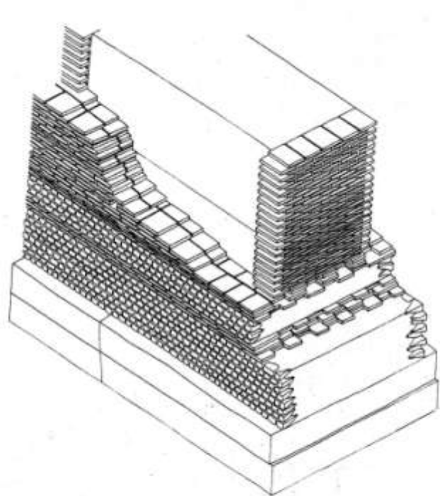
Fig. 15 — Schéma du système d'accrochage des murettes transversales du blocage avec les parements.
